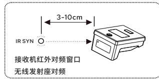
发射座对频窗靠近对接接收机对频灯，完成对频
